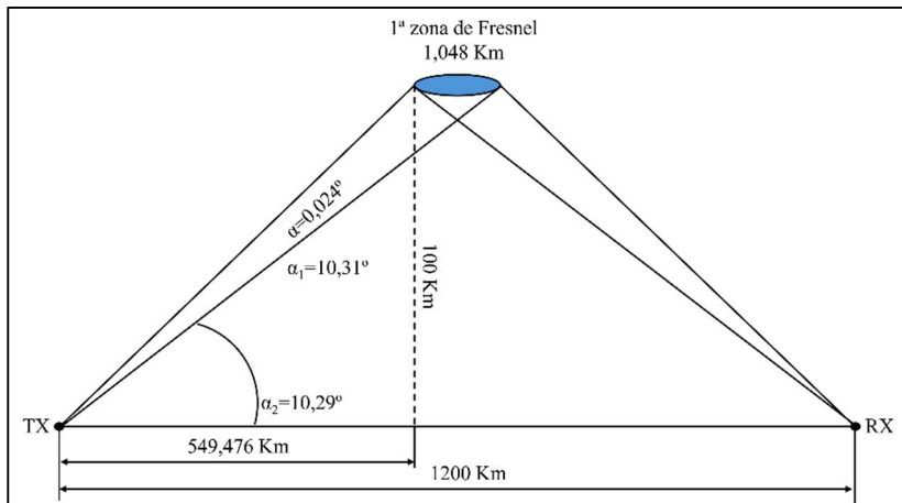
Ilustración 17. Ángulo necesario para iluminar la 1ª zona de Fresnel.
