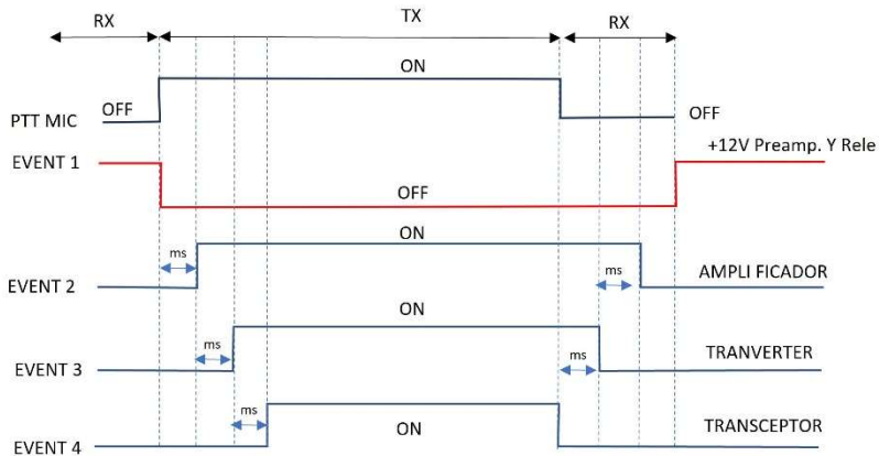
Ilustración 30. Diagrama de tiempos y secuencia normal de conmutación del secuenciador de mi estación.
