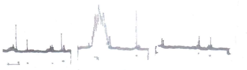
Ilustración 39. Registro real en papel térmico de señales de telegrafía (CW) por reflexión meteórica en 144.100 MHz.
