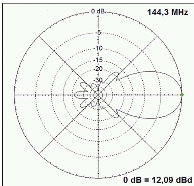
Ilustración 27. Lóbulo de radiación horizontal típico de una antena Yagi de 9 elementos para la banda de 2 metros.
