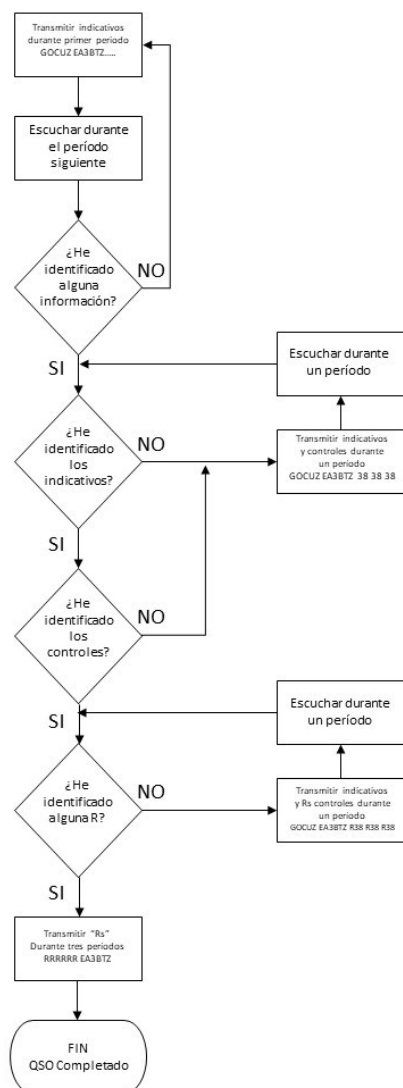
Ilustración 24. Diagrama realización QSO en Meteor Scatter
