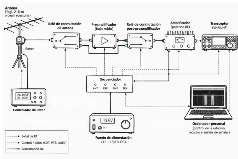
Ilustración 26 Diagrama de bloques y esquema de conexionado de una estación estándar de VHF optimizada para Meteor Scatter.
