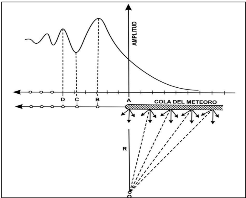
Ilustración 18. Variación de nivel de señal de una reflexión Meteor Scatter.
