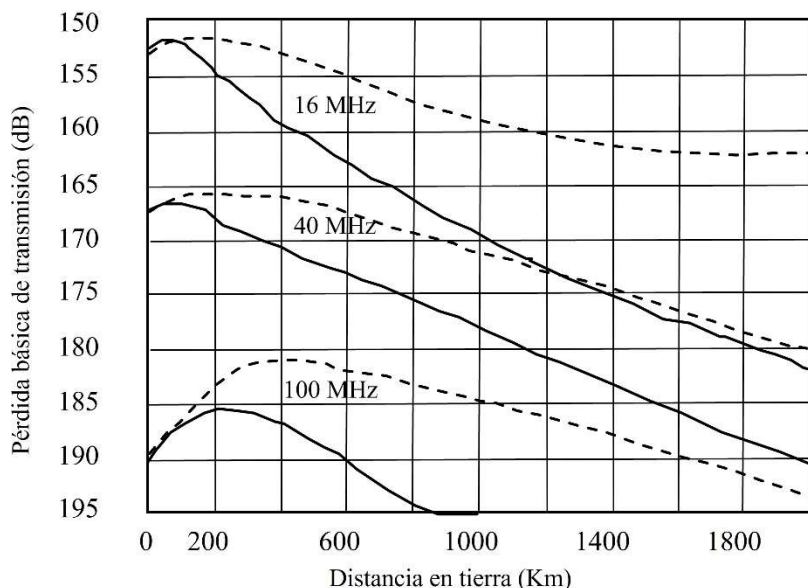
Ilustración 22. Perdida básica de transmisión a diferentes frecuencias
