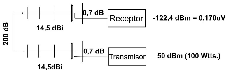
Ilustración 29. Gráfica y desglose del cálculo de nivel de la señal recibida en el extremo remoto.
