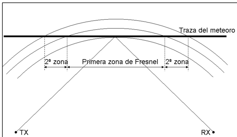
Ilustración 16. Zonas de Fresnel en una geometría de reflexión de meteoros.
