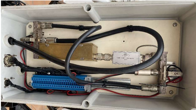
Ilustración 28. Vista interna de la caja estanca con el preamplificador de mástil y los relés de conmutación utilizados por el autor en su estación durante muchos años.
