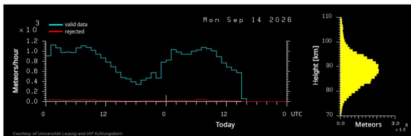
Ilustración 35. Ventana de análisis gráfico de impactos y distribución por altitudes en el software de radio-observación SWAN.
