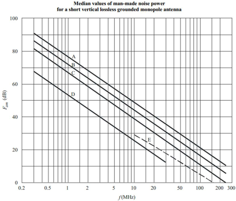
Ilustración 25. Valores de la potencia de ruido equivalente en diferentes entornos en función de la frecuencia.
