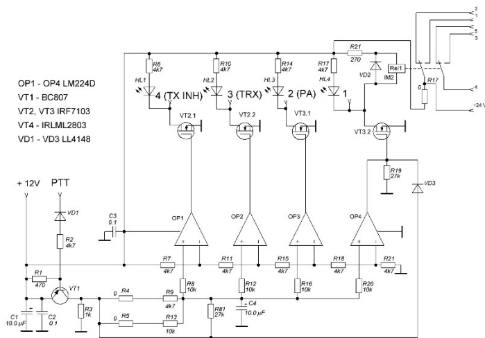
Ilustración 31. Esquema eléctrico de bloques de un secuenciador de cuatro canales de diseño de aficionado.
