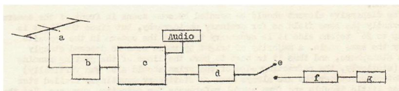
Ilustración 37. Diagrama de bloques del observatorio de radio analógico propuesto originalmente por la BMS.
