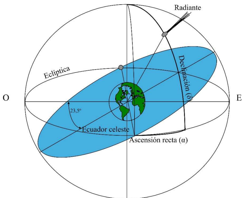
Ilustración 13, Localización de un radiante respecto a la posición de un observador
