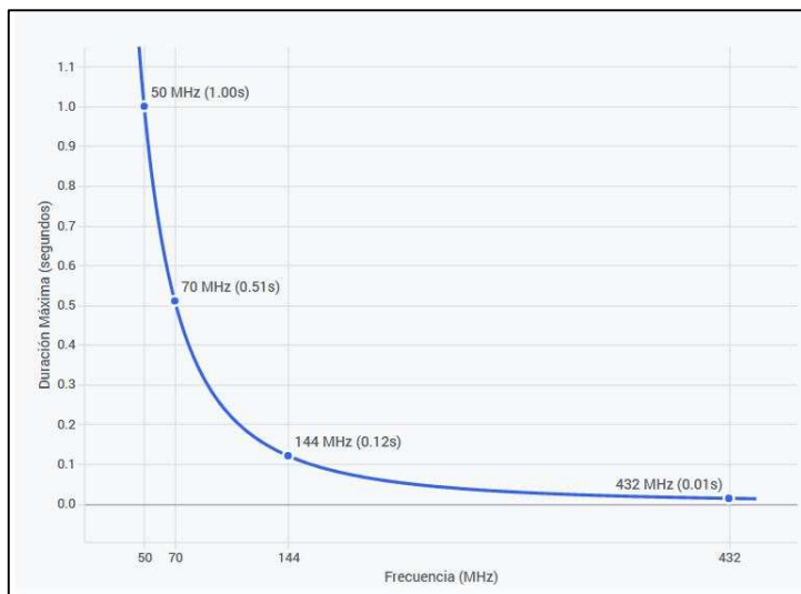
Ilustración 15. Duración máxima teórica de una reflexión subdensa en función de la frecuencia de trabajo.
