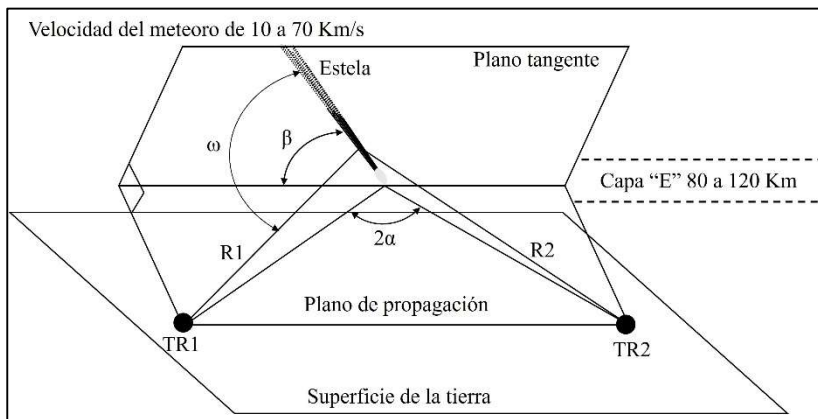
Ilustración 19. Geometría de una traza meteórica
