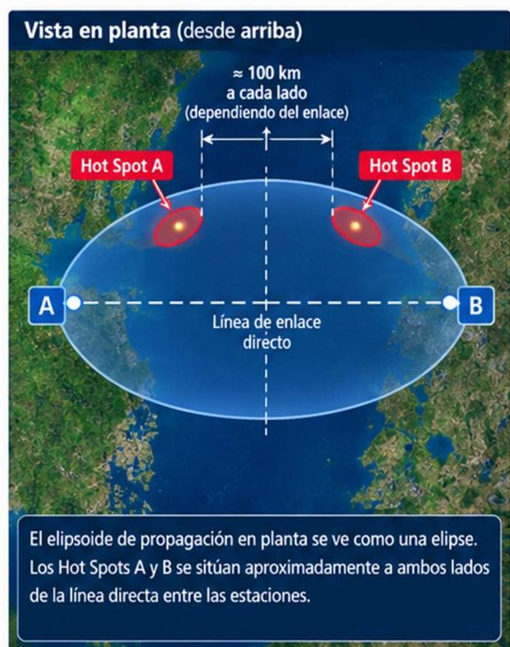
Ilustración 46. Vista en planta del elipsoide de propagación y localización geométrica de los dos Hot Spots laterales (puntos calientes A y B).
